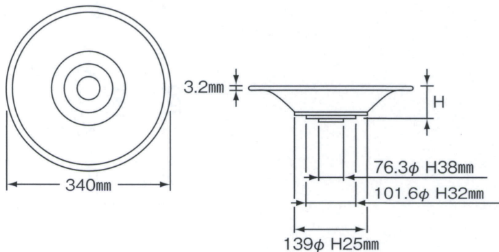
No.112 340mmφ ラッパ型6ヶ穴 ノックダウン受座 76.3φ、101.6φ (1.6t)、139φ (2t) パイプ用ボルト式、溶接可 ¥3,150
