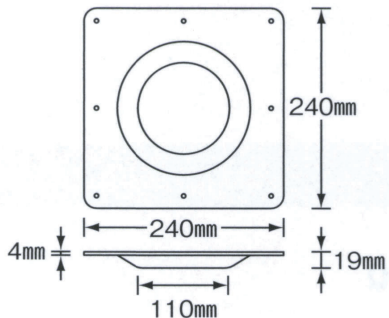
No.116・No.117 240×240 木ネジ8ヶ穴 No.116 ボルト式ノックダウン用受座 60.5φ、76.3φ、101.6φパイプ用 ¥2,050 No.117 溶接用受座 ¥1,350
