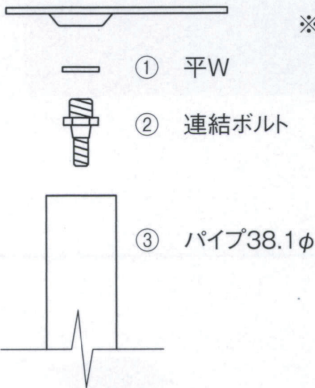
<組立図>
