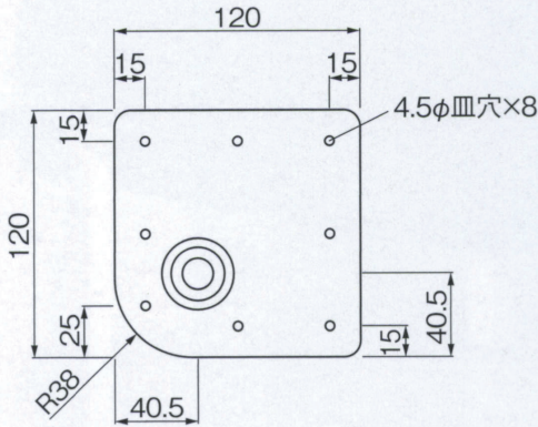
<組立図>
